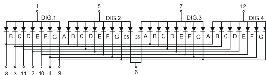
FYQ-4044Bx
